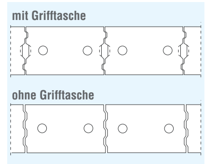
KS-Mauerwerk ohne Stoßfugenvermörtelung (Draufsicht)
