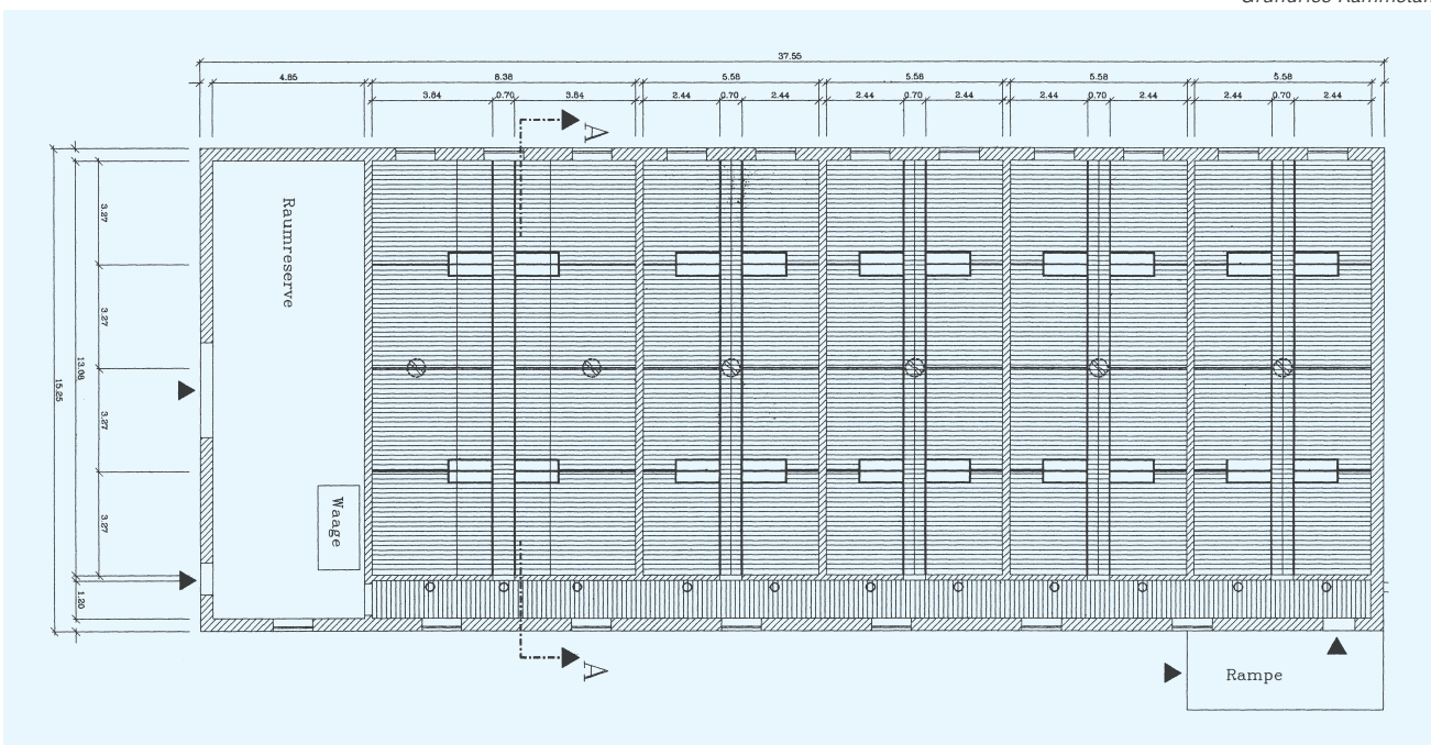
Grundriss Kammstall
